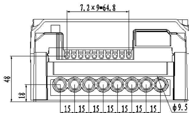
а) Клеммная колодка счетчика РОТЕК РТМ-03(D1) прямого включения
