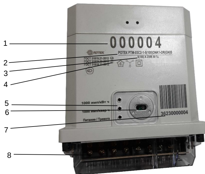
Рисунок 6.1. Внешний вид счетчика РТМ-03(С2) в сплит-исполнении.
