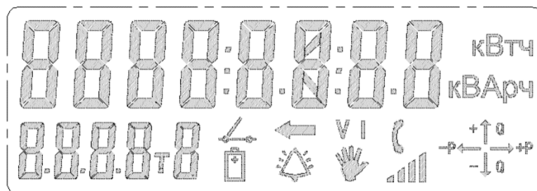
Рисунок 5.5. Символы LCD дисплея счетчика РОТЕК РТМ-03(С1)
