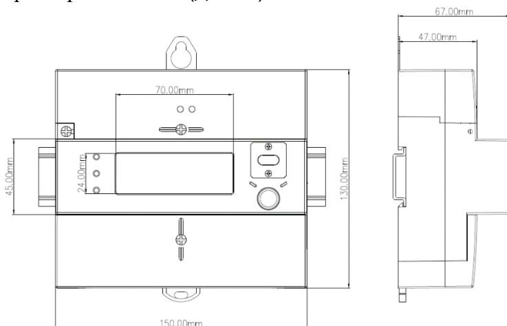
Рисунок 4.5. Габаритные размеры счетчика РОТЕК РТМ-03(В1).
