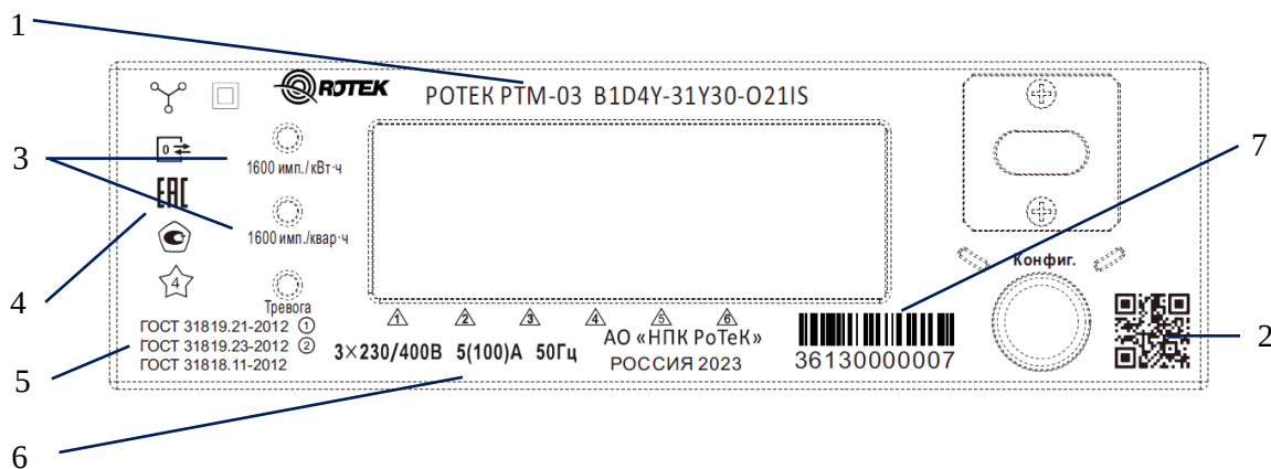
Рисунок 4.3. Обозначения на лицевой панели счетчика РОТЕК РТМ-03(В1)
