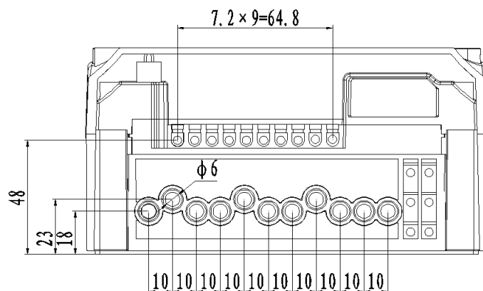
Рисунок 3.4. Расположение и размеры клемм для счетчиков РОТЕК РТМ-03(D1) прямого (а) и трансформаторного (б) включения
