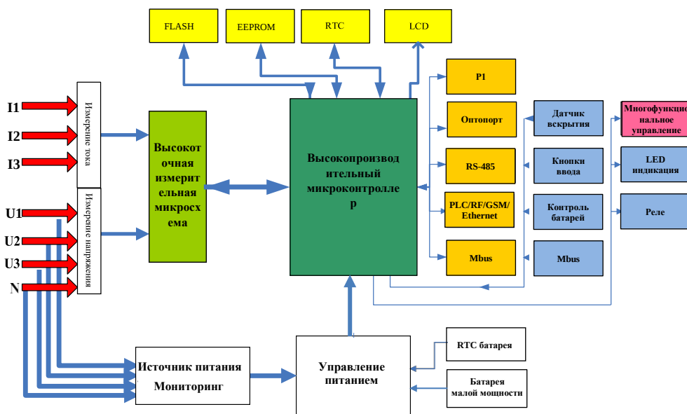
Рисунок 1.2 Блок-схема счетчика POTEK PTM-03
