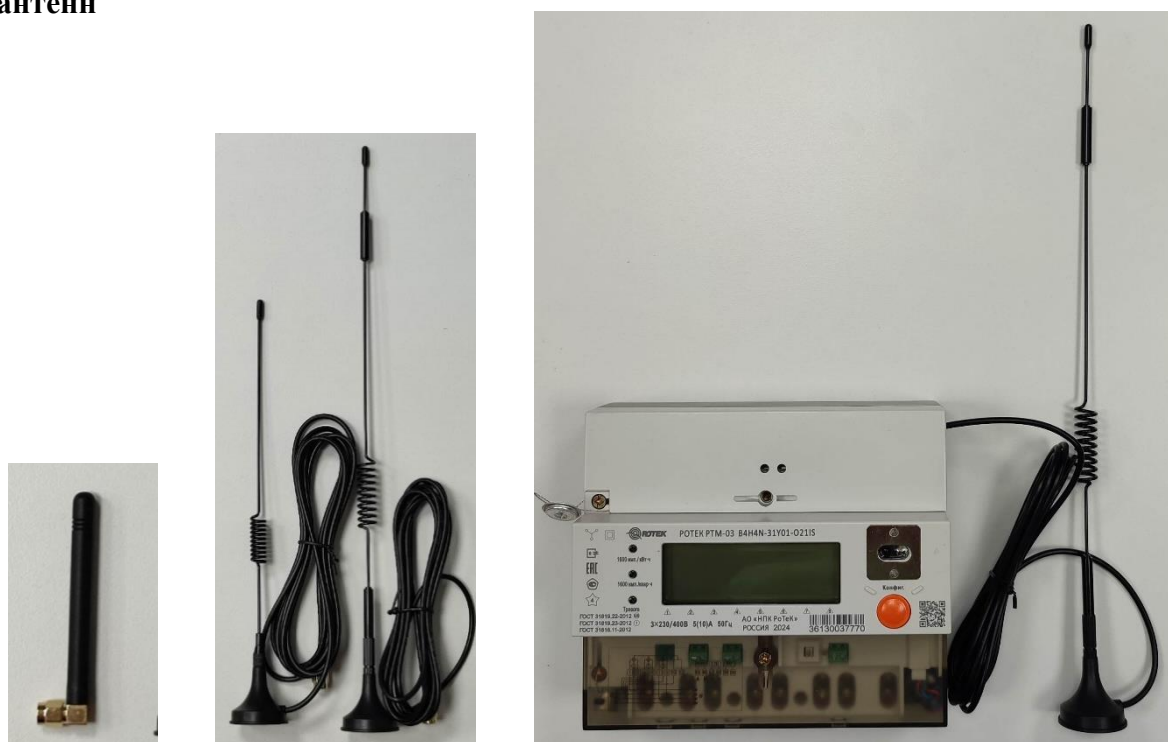
а) Внутренняя антенна б) Внешние антенны в) ПУ РТМ-03(В1) с внешней антенной.
