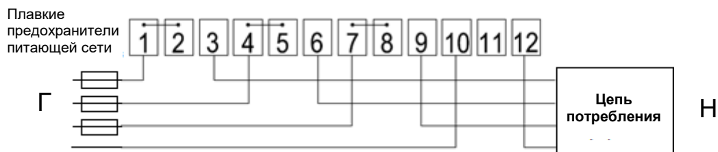
Рисунок 7.1-1. Подключение счетчика прямого включения к фазным проводам и проводу нейтрали
