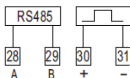
Рисунок 3.6. Схема подключения интерфейсных контактов счетчиков ПОТЕК РТМ-03(D1) прямого включения.
