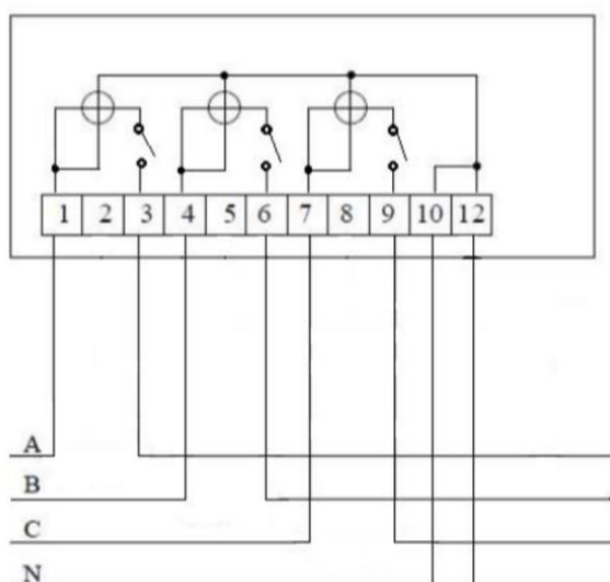
Рисунок 6.3. Схема подключения счетчика к силовой сети
