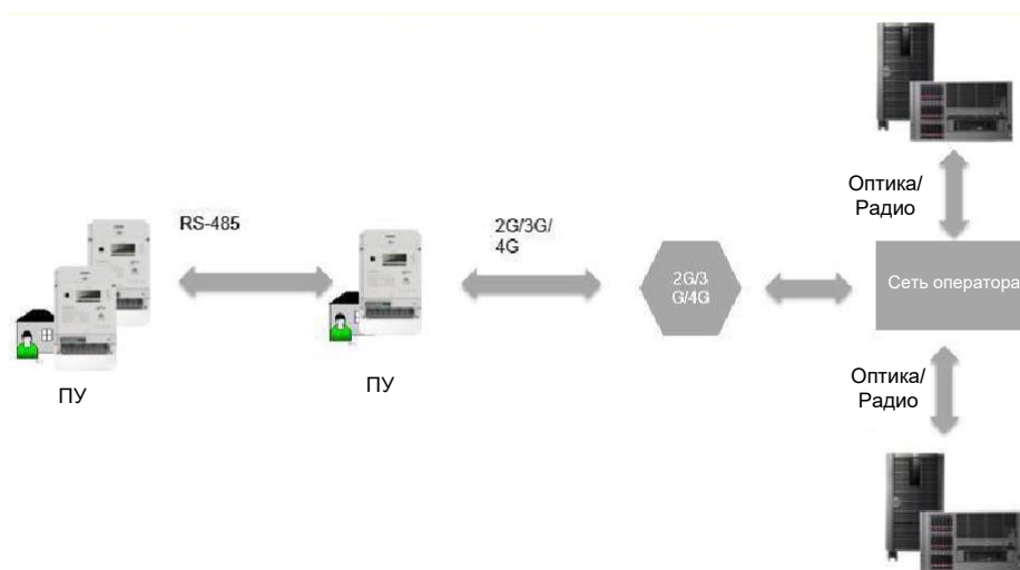
Рисунок 8.1 Схема ретрансляции
