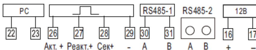
Рисунок 3.7. Схема подключения сигнальных цепей счетчиков ПОТЕК РТМ-03(D1) трансформаторного включения с двумя интерфейсами RS-485 и входом внешнего резервного питания 1 .
