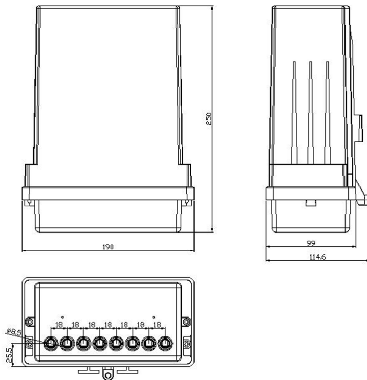
Рисунок 5.6. Размеры счетчика РОТЕК РТМ-03(С1)
