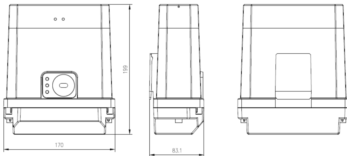
Рисунок 6.6. Размеры счетчика РОТЕК РТМ-03(С2)
