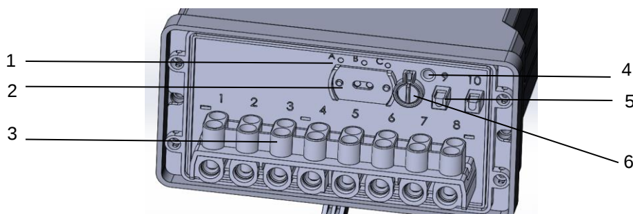
Рисунок 5.2. Расположение выводов и контактов счетчика РТМ-03(С1) в сплит-исполнении.
