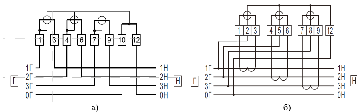
Рисунок 4.7. Схемы подключения к силовой сети счетчиков РОТЕК РТМ-03(В1) прямого включения (а) и трансформаторного включения через ТТ (б).
