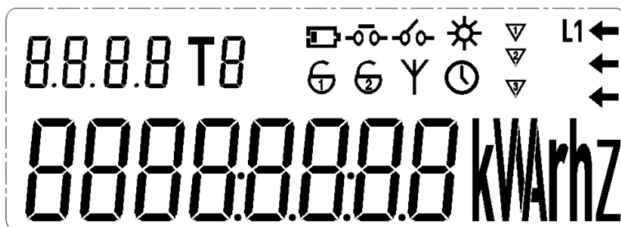
Рисунок 6.5. Символы LCD дисплея счетчика РОТЕК РТМ-03(С2)
