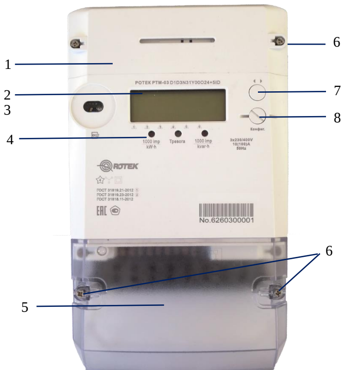
Рисунок 3.1 Счетчик РТМ-03(D1) в сборе с прозрачной терминальной крышкой
