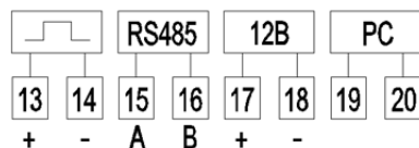
Рисунок 4.4. Схема подключения сигнальных цепей счетчиков РОТЕК РТМ-03(В1) со входом внешнего резервного питания (опция) 1
