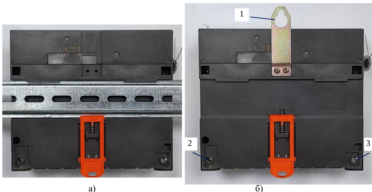
Рисунок 7.5. Крепление счетчика РТМ-03(В1) на DIN-рейку (а) и на 3 точки (б).
