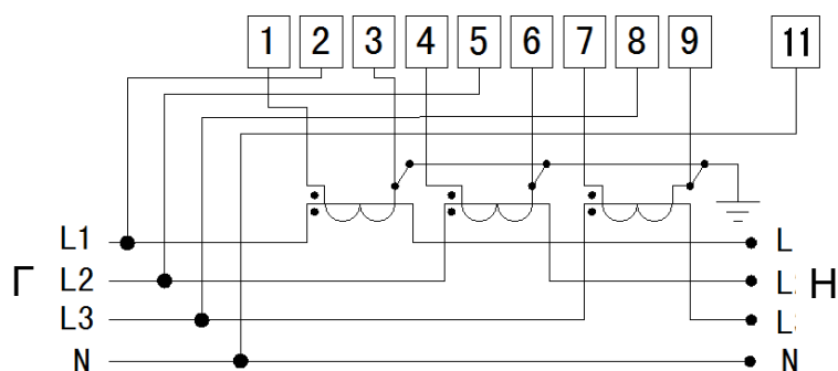
Рисунок 7.1-2. Подключение счетчика трансформаторного включения к фазным проводам и проводу нейтрали
